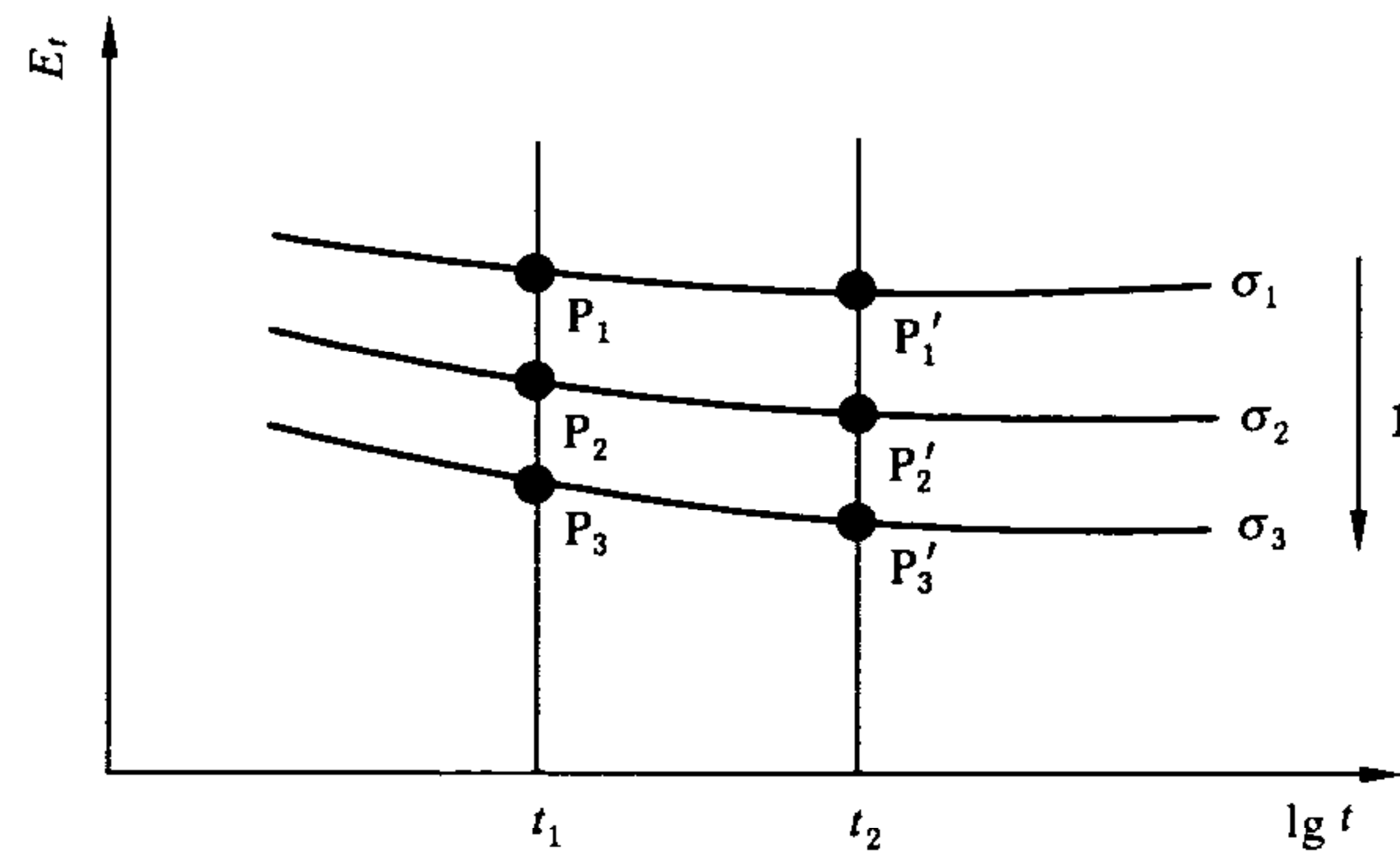
图 2 蠕变模量-时间曲线
