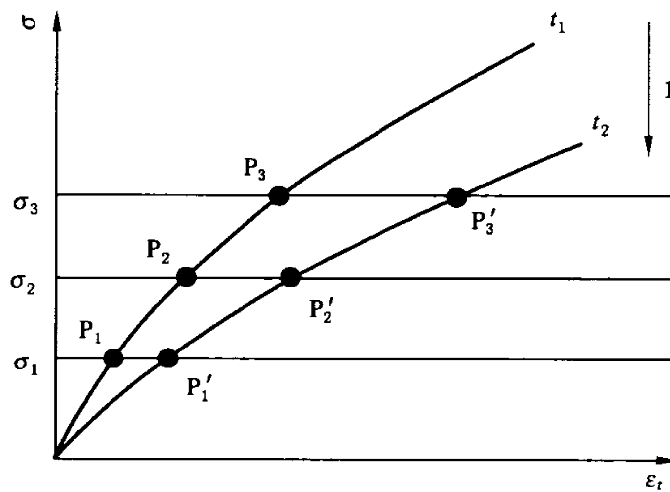
图 3 等时应力-应变曲线
